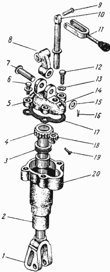
Рис. 61. Регулируемый раскос
